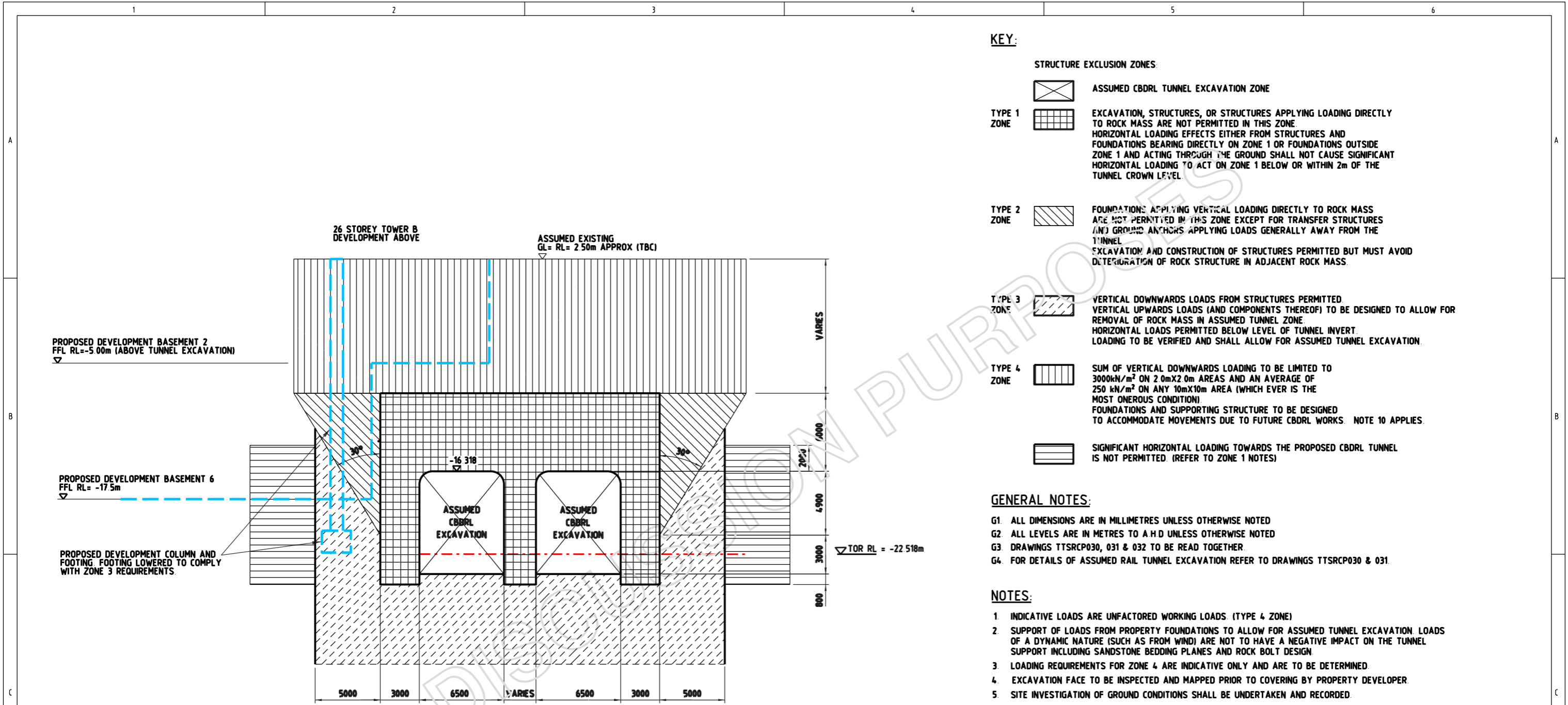
SECTION A-A
